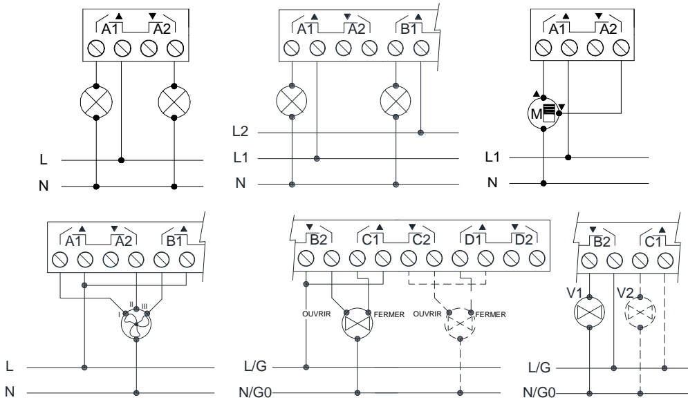
Figure 2: Exemples de connexions (de gauche à droite et de haut en bas): 2 charges, 2 charges avec phases différentes, volet roulant, ventilo convecteur avec 3 vitesses, vannes de ventilo convecteur de trois points et vannes de ventilo convecteur tout ou rien.
