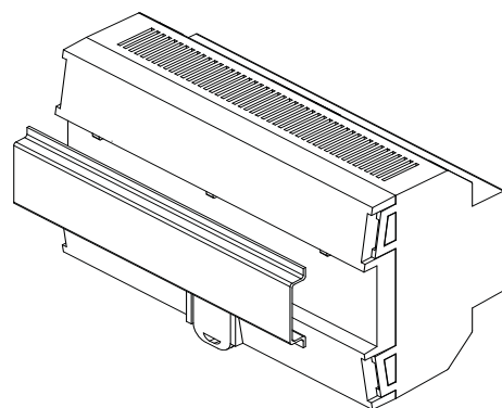
Figure 3: Montage du MINiBOX QUATRO sur rail DIN
