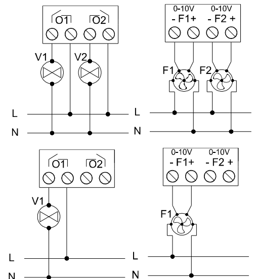
Figure 2: (de haut en bas et de gauche à droite) Exemple de connexions dans le bloc de sorties individuelles 1 et de sorties 0 - 10VDC de deux vannes, deux ventilateurs, une vanne et un ventilateur.
