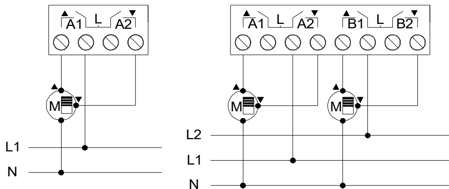
Figure 3: Exemple de connexion (de gauche à droite): un volet dans le canal A et deux volets dans les canaux A et B avec des phases différentes.
