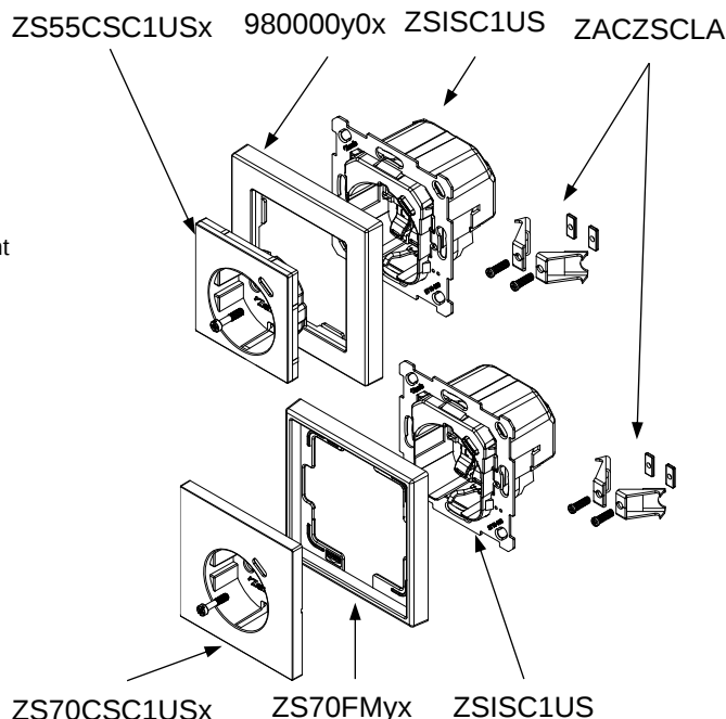
Figure 1. Base de prise Schuko avec USB type C.
