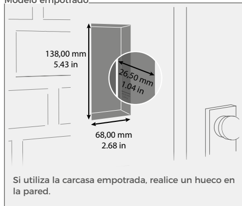
Modelo empotrado
